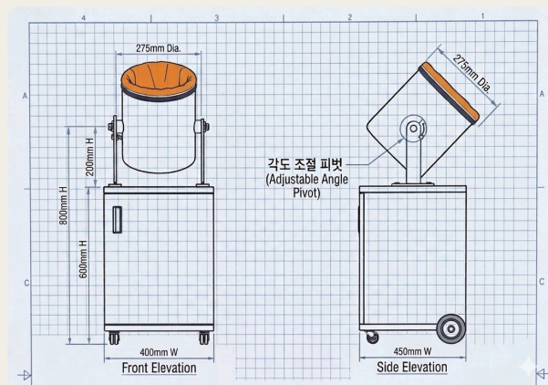
• 장비 정면도, 측면도
