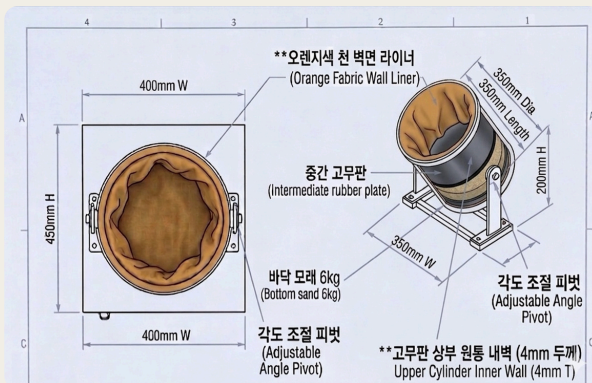
• 입구 평면도, 장비 조감도
